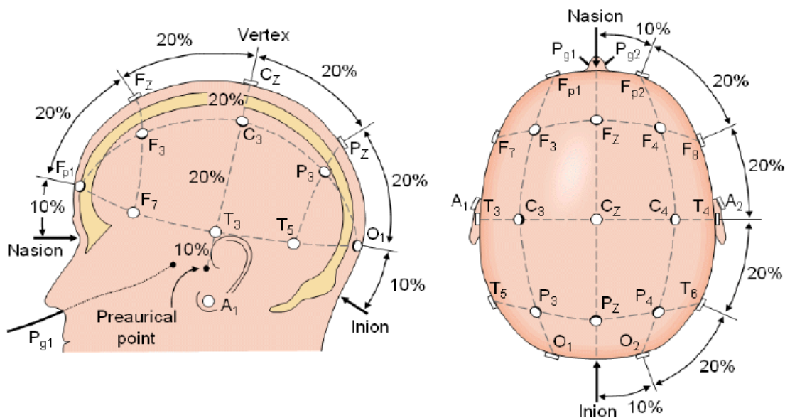
Figura 3: Sistema internacional 10-20
