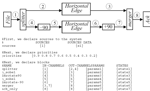
Fig. 2. (arriba) Ejemplo de diagrama de módulos de un sistema AER. (abajo) Fichero Netlist que lo describe.
