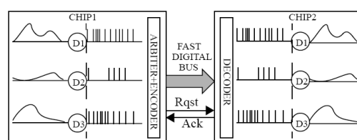
Fig. 1. Enlace de comunicación AER punto a punto
