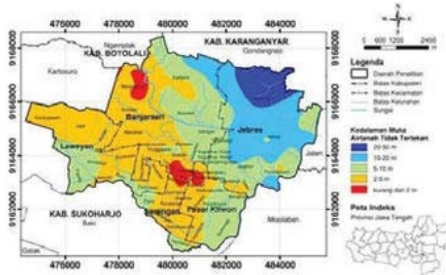
Gambar 5. Peta parameter kedalaman muka airtanah tidak tertekan.
