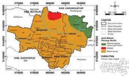
Gambar 4. Peta parameter jenis litologi di atas akuifer.
