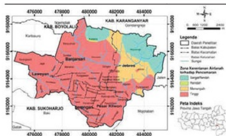
Gambar 6. Peta kerentanan airtanah terhadap pencemaran.
