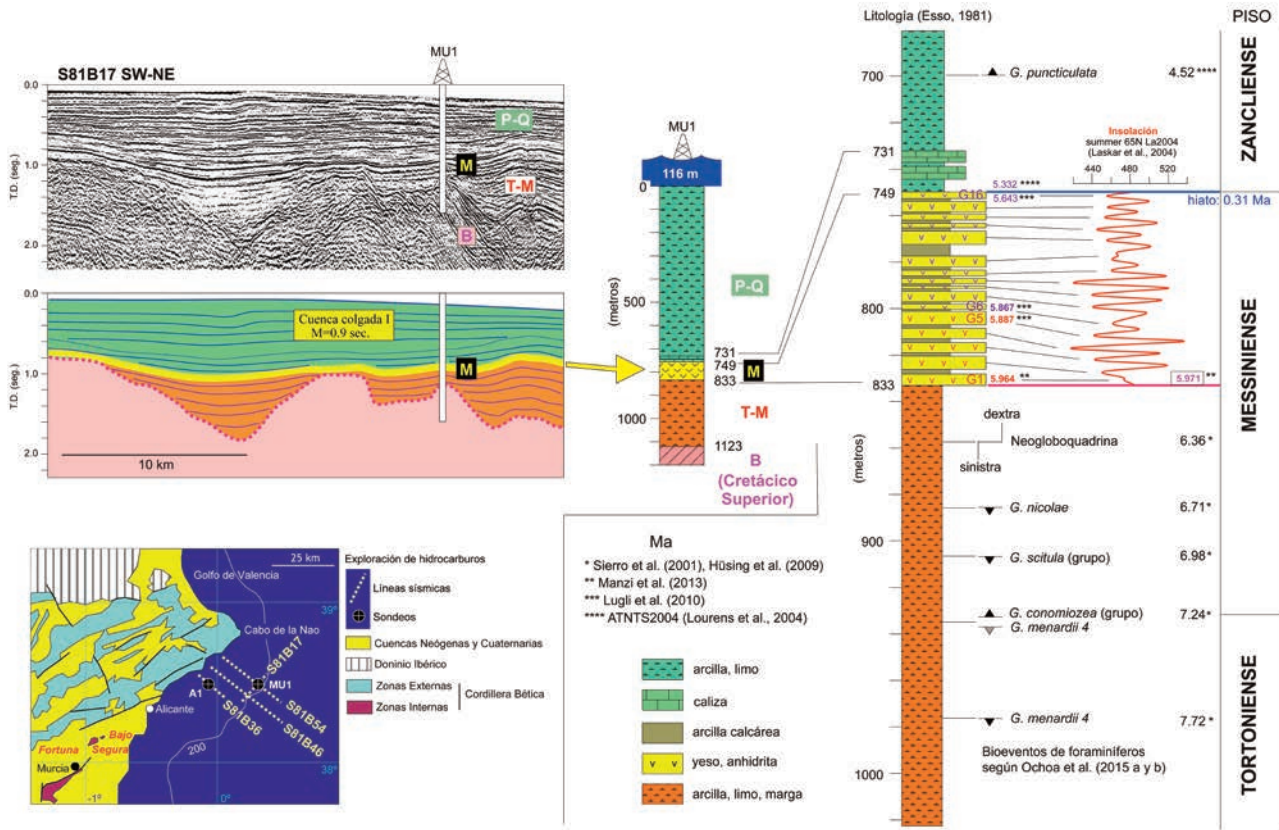
Fig. 2.- Expresión sísmica, litología y calibración temporal del horizonte M (Unidad Evaporítica del Messiniense). Ver referencias para las edades (Ma) de los bioeventos y ciclos de insolución La2004. Ver figura en color en la web.
