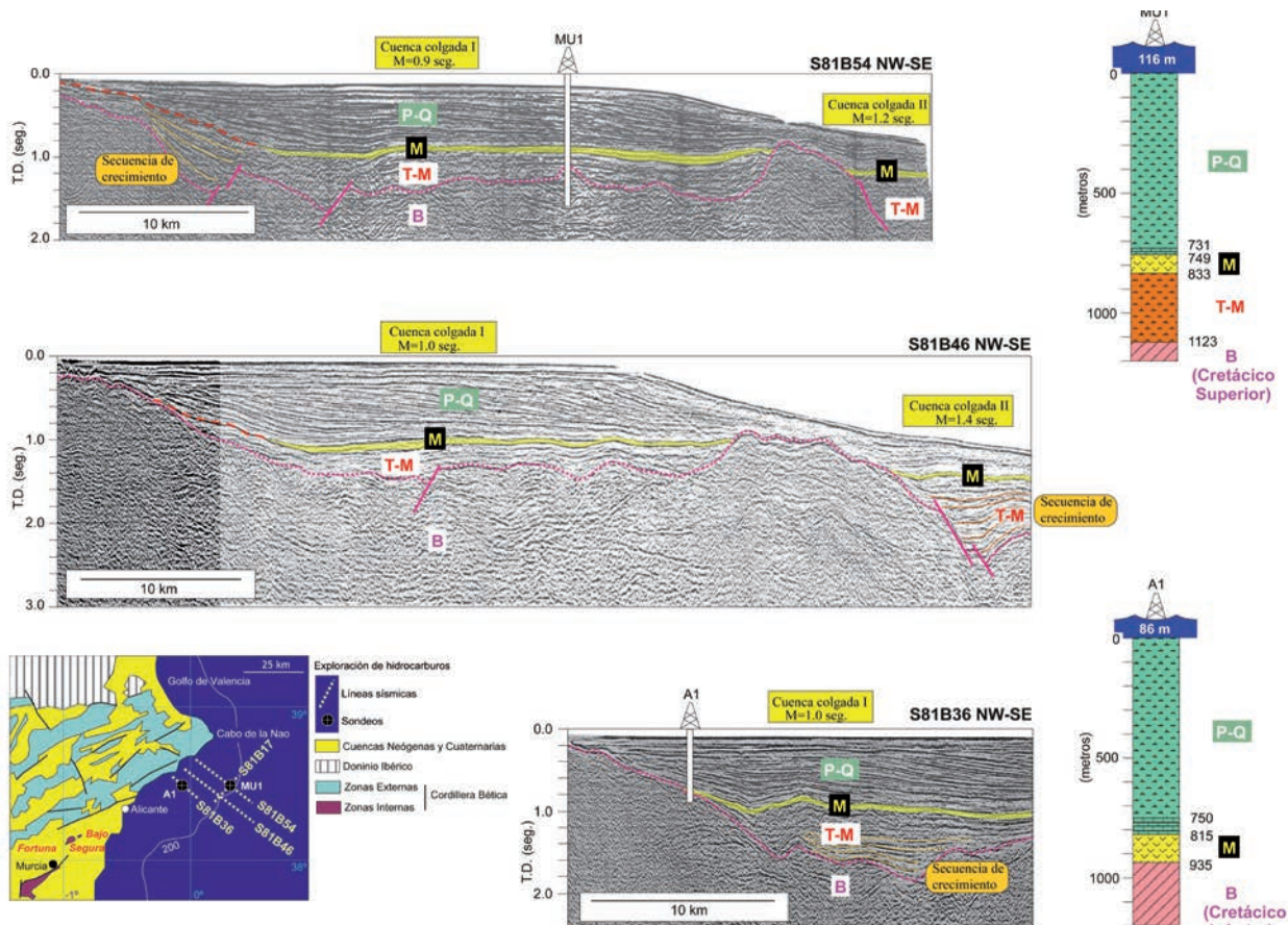
Fig. 1- Unidades litosísmicas reconocidas en la plataforma continental de Alicante a partir de líneas sísmicas (tiempo doble en segundos) y sondeos. Nótese la distribución de la Unidad T-M y el horizonte M en dos cuencas colgadas a diferente batimetría, así como la geometría progradante del prisma sedimentario P-Q. Ver figura en color en la web.
