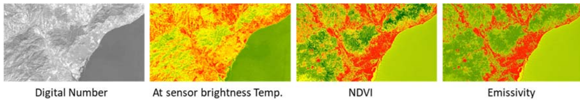
Figure n. 8: LST process
