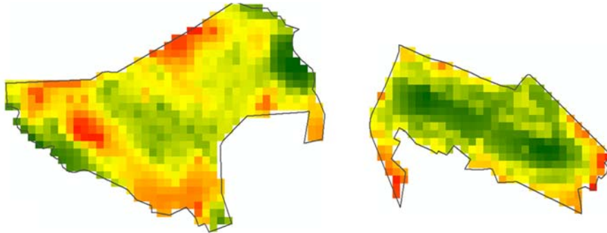
Figure 15. LST (Landsat 8)
