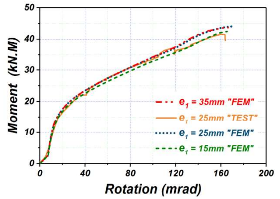
(d) M- \Phi curves for different bolt edge distances e_i
