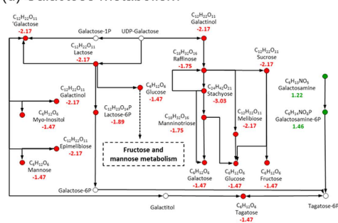
(d) Galactose metabolism
