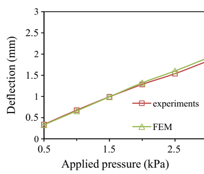
(d) Maximum deflections in VGU panel
