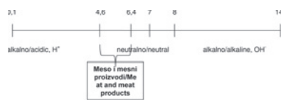
Slika 1. Skala pH vrijednosti Figure 1. pH scale
