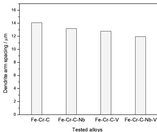
Figure 5: Dendrite arm spacing in the tested alloys Slika 5: Razdalja med dendritnimi vejami v preizkusnih zlitinah
