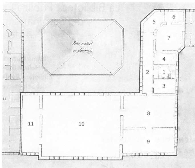
Figura 1. S'indiquen els espais dedicats a la biblioteca segons els plànols del primer projecte del Seminari Conciliar, del 1879 (AHCOAC): (1) escala d'accés a la biblioteca i a l'Observatori de l'Est; (2) galeria pública d'impresos; (3) despatx del bibliotecari; (4) dipòsit de duplicats; (5) arxiu de llibres reservats; (6) restauració de llibres; (7) sala de lectura dels col·legials de l'Institut; (8) sala de lectura pública; (9) sala de lectura per als senyors catedràtics i persones distingides; (10) gran sala de la biblioteca; (11) sala de lectura per a seminaristes.
