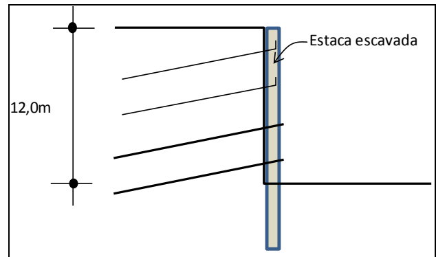
Figura 24. Cortina em estacas escavadas com apoio misto (Caso 2F).
