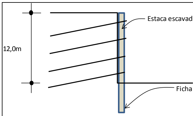
Figura 23. Cortina em estacas escavadas (Caso 2E).
