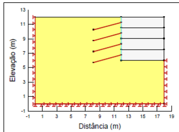
Figura 10. Concepção final do projeto (Caso 1).
