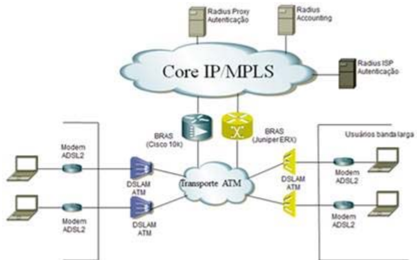
Figura 2: Rede ADSL com transporte ATM
