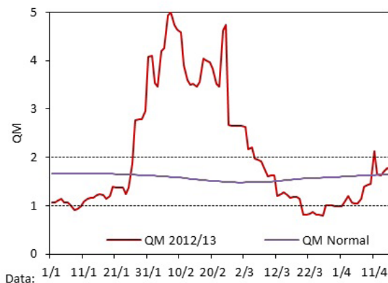
Fig. 4. Temperatura, chuva, insolação, dias de chuva e balanço hídrico de cultivo ( \text{CAD} = 80 \text{ mm} ) e Quociente Heliopluiométrico de Maturação (QM), em Bento Gonçalves , RS, safra 2012/13. Fonte dos dados: Embrapa Uva e Vinho. Abreviações e legenda: Mínima abs: mínima absoluta; Máxima abs: máxima absoluta; Média mín: média das mínimas; Média máx: média das máximas; Insol.: insolação; D.chuva: dias do mês com chuva; ARM: armazenamento hídrico; DEF: deficiência hídrica; EXC: excedente hídrico.
