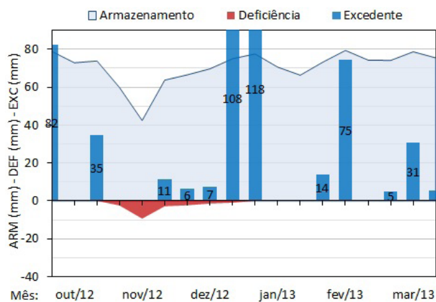
Fig. 5. Temperatura, chuva, insolação, dias de chuva e balanço hídrico de cultivo (CAD = 80 mm) e Quociente Heliopluviométrico de Maturação (QM), em Encruzilhada do Sul, RS, safra 2012/13. Fonte dos dados: INMET. Abreviações e legenda: Mínima abs: mínima absoluta; Máxima abs: máxima absoluta; Média mín: média das mínimas; Média máx: média das máximas; Insol.: insolação; D. chuva: dias do mês com chuva; ARM: armazenamento hídrico; DEF: deficiência hídrica; EXC: excedente hídrico.
