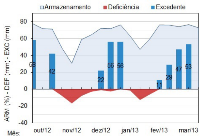
Fig. 3. Temperatura, chuva, insolação, dias de chuva e balanço hídrico de cultivo (CAD = 80 mm) e Quociente Heliopluiométrico de Maturação (QM), em Vacaria, RS, safra 2012/13. Fonte dos dados: INMET e Embrapa Uva e Vinho. Abreviações e legenda: Mínima abs: mínima absoluta; Máxima abs: máxima absoluta; Média mín: média das mínimas; Média máx: média das máximas; Insol.: insolação; D. chuva: dias do mês com chuva; ARM: armazenamento hídrico; DEF: deficiência hídrica; EXC: excedente hídrico.
