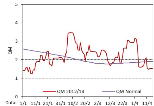
Fig. 6. Temperatura, chuva, insolação, dias de chuva e balanço hídrico de cultivo (CAD = 60 mm) e Quociente Heliopluiométrico de Maturação (QM), em Santana do Livramento, RS, safra 2012/13. Fonte dos dados: INMET. Abreviações e legenda: Mínima abs: mínima absoluta; Máxima abs: máxima absoluta; Média mín: média das mínimas; Média máx: média das máximas; Insol.: insolação; D. chuva: dias do mês com chuva; ARM: armazenamento hídrico; DEF: deficiência hídrica; EXC: excedente hídrico.
