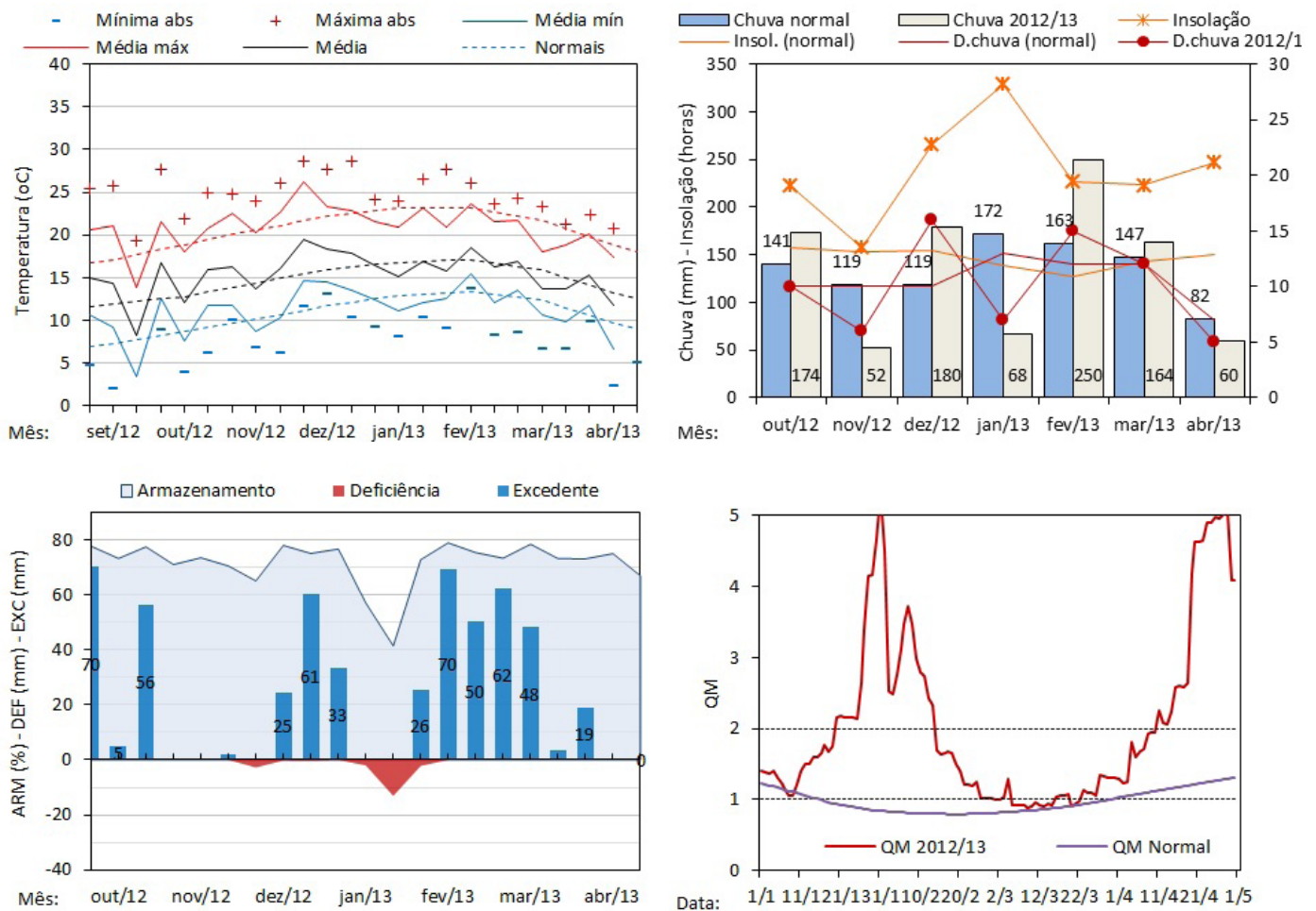
Fig. 2. Temperatura, chuva, insolação, dias de chuva e balanço hídrico de cultivo (CAD = 80 mm) e Quociente Heliopluiométrico de Maturação (QM), em São Joaquim, SC, safra 2012/13. Fonte dos dados: INMET e Embrapa Uva e Vinho. Abreviações e legenda: Mínima abs: mínima absoluta; Máxima abs: máxima absoluta; Média mín: média das mínimas; Média máx: média das máximas; Insol.: insolação; D. chuva: dias do mês com chuva; ARM: armazenamento hídrico; DEF: deficiência hídrica; EXC: excedente hídrico.
