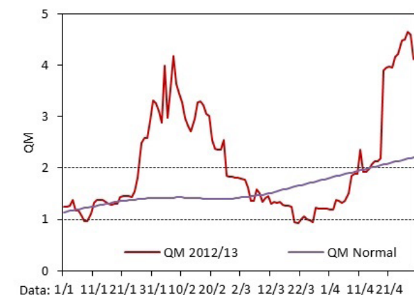
Fig. 3. Temperatura, chuva, insolação, dias de chuva e balanço hídrico de cultivo (CAD = 80 mm) e Quociente Heliopluiométrico de Maturação (QM), em Vacaria, RS, safra 2012/13. Fonte dos dados: INMET e Embrapa Uva e Vinho. Abreviações e legenda: Mínima abs: mínima absoluta; Máxima abs: máxima absoluta; Média mín: média das mínimas; Média máx: média das máximas; Insol.: insolação; D. chuva: dias do mês com chuva; ARM: armazenamento hídrico; DEF: deficiência hídrica; EXC: excedente hídrico.
