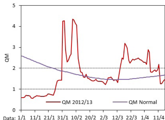
Fig. 5. Temperatura, chuva, insolação, dias de chuva e balanço hídrico de cultivo (CAD = 80 mm) e Quociente Heliopluviométrico de Maturação (QM), em Encruzilhada do Sul, RS, safra 2012/13. Fonte dos dados: INMET. Abreviações e legenda: Mínima abs: mínima absoluta; Máxima abs: máxima absoluta; Média mín: média das mínimas; Média máx: média das máximas; Insol.: insolação; D. chuva: dias do mês com chuva; ARM: armazenamento hídrico; DEF: deficiência hídrica; EXC: excedente hídrico.
