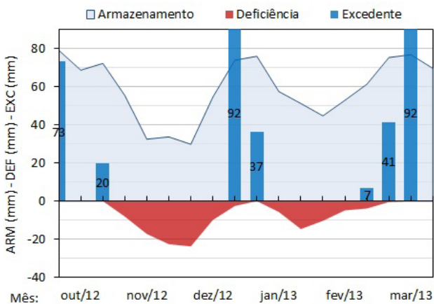
Fig. 4. Temperatura, chuva, insolação, dias de chuva e balanço hídrico de cultivo ( \text{CAD} = 80 \text{ mm} ) e Quociente Heliopluiométrico de Maturação (QM), em Bento Gonçalves , RS, safra 2012/13. Fonte dos dados: Embrapa Uva e Vinho. Abreviações e legenda: Mínima abs: mínima absoluta; Máxima abs: máxima absoluta; Média mín: média das mínimas; Média máx: média das máximas; Insol.: insolação; D.chuva: dias do mês com chuva; ARM: armazenamento hídrico; DEF: deficiência hídrica; EXC: excedente hídrico.
