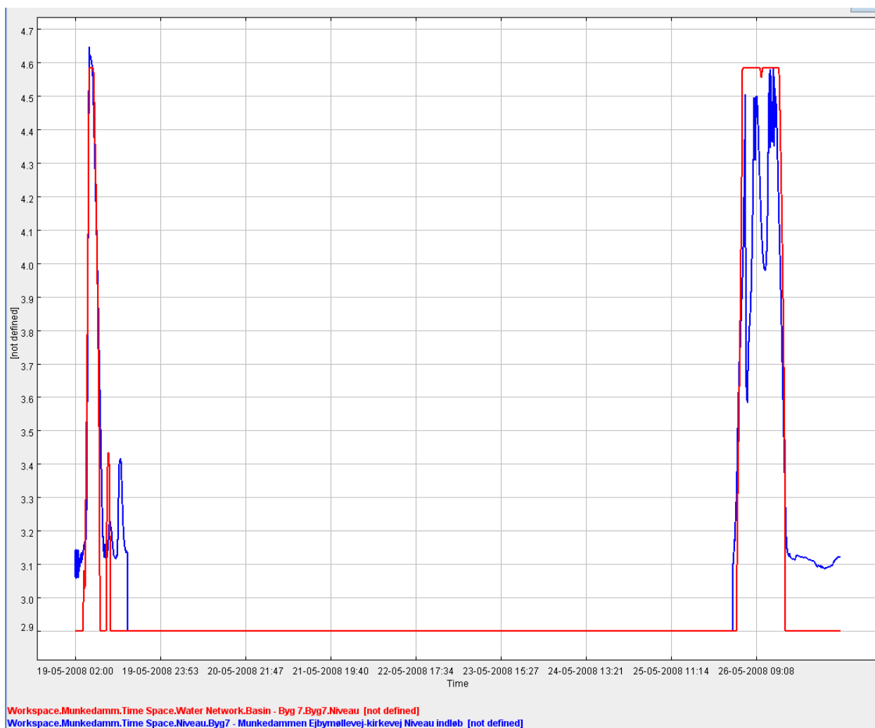
Figur 6.6.2.c Målt og modelleret niveau i bygværk 7 i Munkedammen bassinledning. Den blå linje er det målte.
