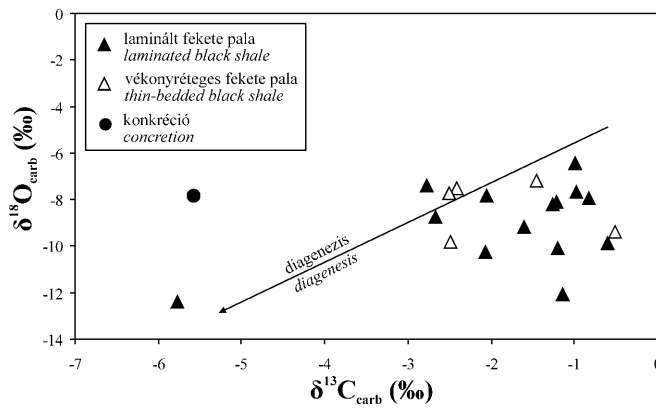
8. ábra. A karbonát stabilizotópos összetétele: \delta^{13}\text{C}_{\text{carb}} (V-PDB)– \delta^{18}\text{O}_{\text{carb}} (V-PDB) diagram
