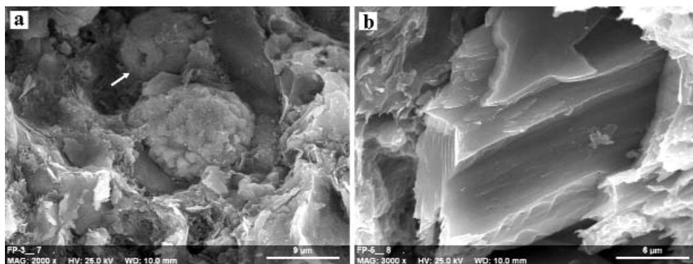
7. ábra. Az Óbányai Aleurolit Formáció karbonátjának szekunder elektronképei (SEI). a) framboidális pirít, ami gyakran üres Schizosphaerella vázat tölt ki, a háttérben szétesett schizospherák láthatók (nyíl); b) pátos biokaszt- vagy cementtöredék
