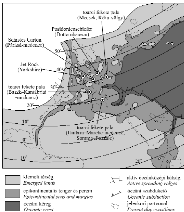
1. ábra. A vizsgált terület ösföldrajzi kerete (BASSOUILLET et al. 1993), valamint néhány alsó-toarci fekete pala rétegsor helyzete (JENKYN 1985, 1988)
