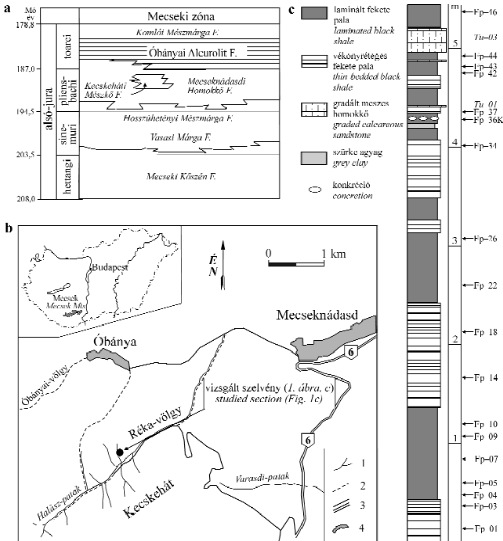
2. ábra. a) A Mecseki zóna alsó-jura formációinak rétegtani helyzete (HAAS 1994); b) A vizsgált szelvény földrajzi elhelyezkedése. 1: patak; 2: turistaút; 3: műút; 4: település; c) Az alsó-toarci fekete pala (Óbányai Aleurolit Formáció) Réka-völgyi szelvényének egyszerűsített rétegsora a mintavételi pontok feltüntetésével (alsó rész)
