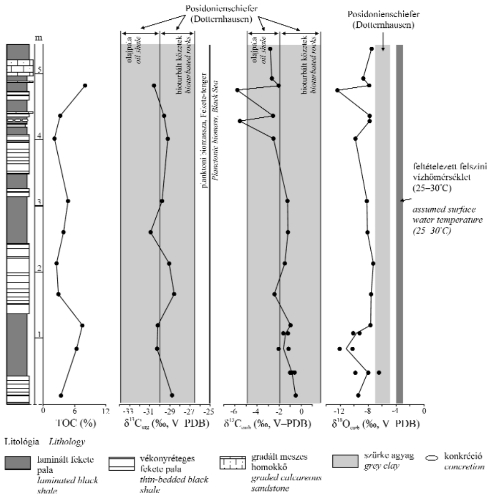
6. ábra. A TOC, a \delta^{13}C és a \delta^{18}O adatok változása az Óbányai Aleurolit Réka-völgyi szelvényében (Mecsek hegység). A feltüntetett további adatok: Posidonienschiefer, alsó-toarci, Dotternhausen (SCHMID-RÖHL 1999; RÖHL et al. 2001); fekete-tengeri plankton biomassza FREEMAN et al. (1994) alapján; feltételezett trópusi-szubtrópusi felszíni vízhőmérséklet SCHMID-RÖHL (1999) és RÖHL et al. (2001) alapján
