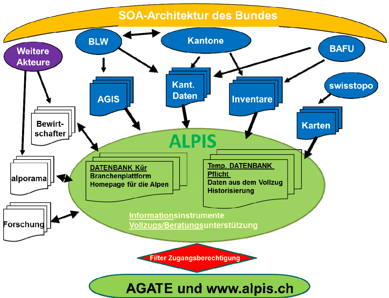
Abbildung 2: . ALPIS soll in die Service Orientiert Architektur – SOA des BLW integriert werden und Daten aus dem Sömmerungsgebiet liefern und von andern Stellen beziehen können. Die Abbildung zeigt nicht alle möglichen Datenflüsse auf. Pflichtdaten kommen von den Kantonen. Kürdaten kommen von verschiedenen Seiten. Je nach Zugangsberechtigung kann über ALPIS auf Daten der einzelnen Ursprungs-Datenbanken direkt zugegriffen werden
