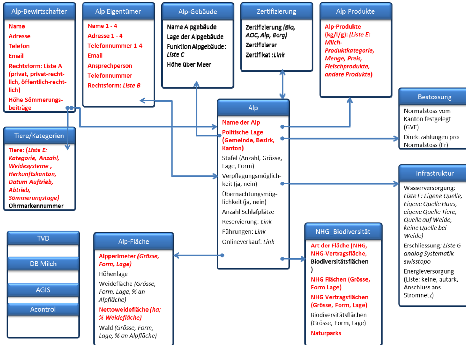
Abbildung 4: Entwurf der Datenbankstruktur von ALPIS. Rot sind die Daten dargestellt, die zum minimalen Datenset gehören. Schwarz die Kürdaten.
