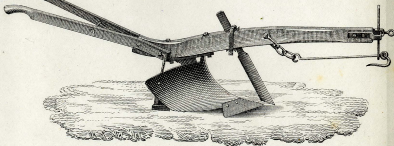
Der Grignon-Pflug als Schwing-Pflug.
