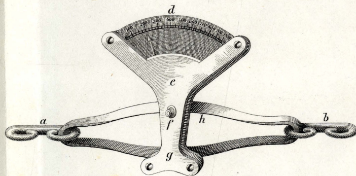
Der Kraftmesser.
