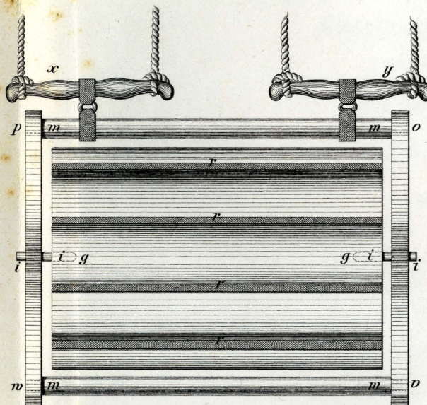
Längensansicht.
