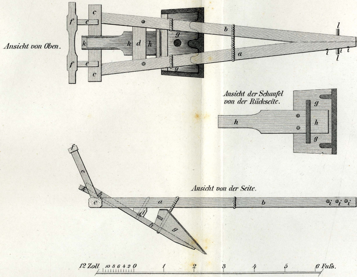
Fig. 2. Der Schaufelpflug.
