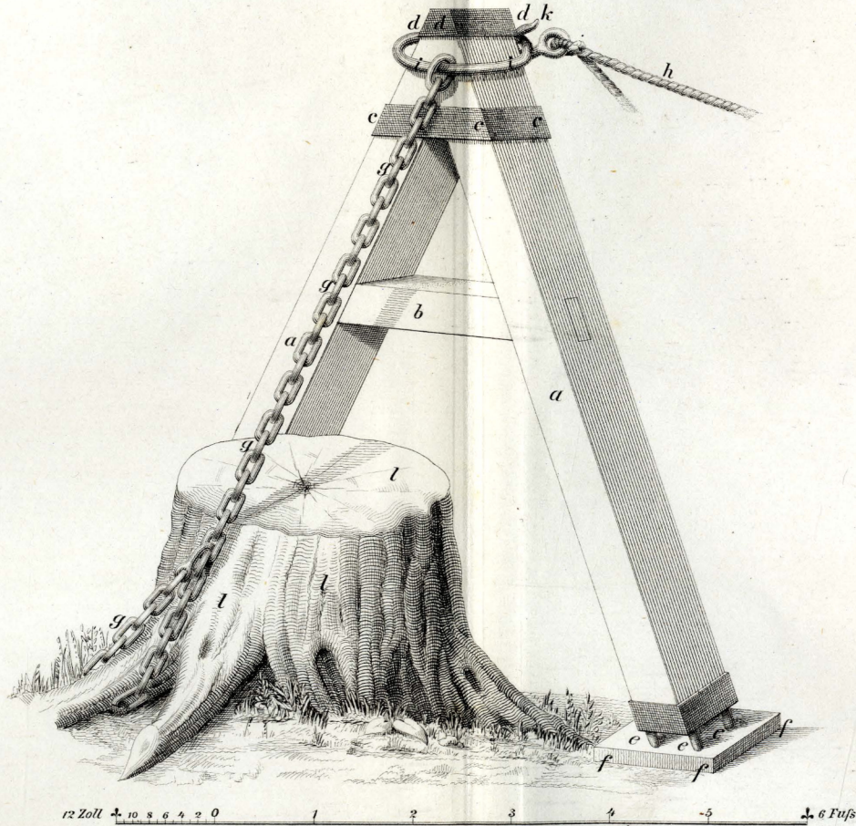
Fig. 3. Apparat zum Ausheben der Baumstubben.
