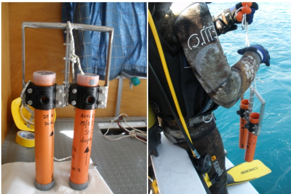
Fig. 3: Doppio carotatore di sedimenti impiegato nella campagna di Giugno 2012.
