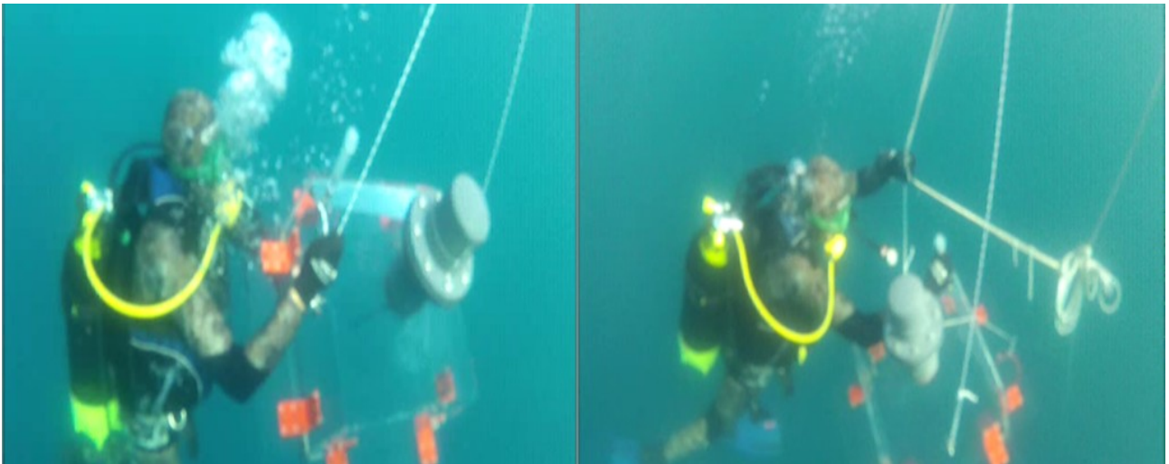
Fig. 7: Posizionamento della camera bentica sul fondo marino per il campionamento dell'acqua all'interfaccia acqua-sedimento (foto subacquee)
