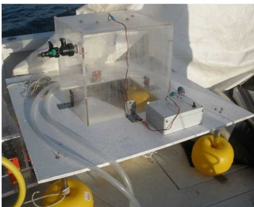
Fig. 8: Camera d'accumulo utilizzata per lo studio dei flussi all'interfaccia acqua- atmosfera.
