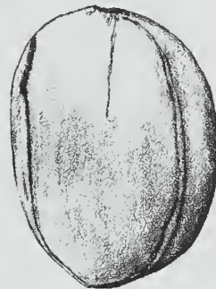
Trigonocarpus parkinsonii X1.25
