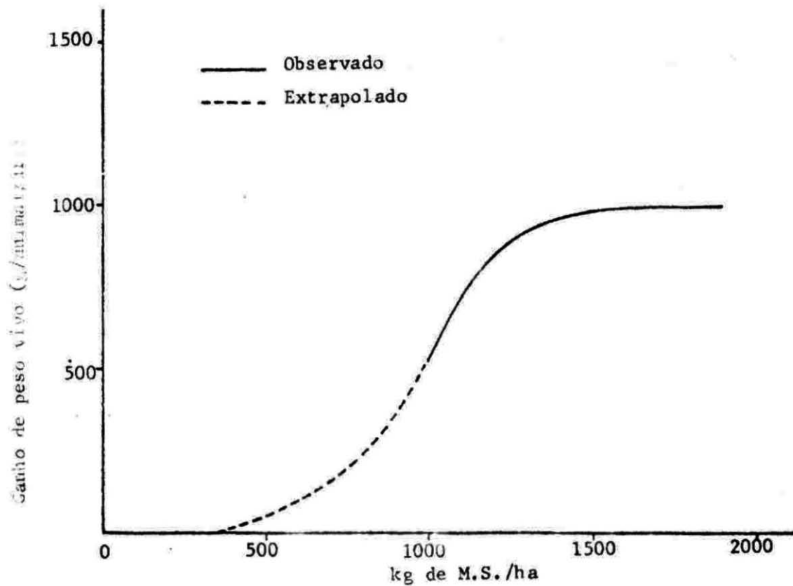
FIGURA 1 - Relação entre a disponibilidade de matéria seca de aveia, e o ganho de peso vivo de animais de sobreano, durante 84 dias de pastejo. 51
