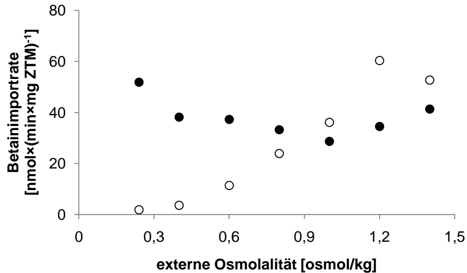
Abbildung 3.13: Einfluss von TC auf die BetP-Transportaktivität in K^+ -vorbeladenen C. glutamicum DHPF (pBetP)-Zellen. Die Zellen wurden vor der Zugabe von 0,25 mM [ ^{14}C ]-Betain 3 min bei 0,8 mM TC (●) oder ohne TC (○) inkubiert. Externer Puffer: 0,1 M NaCl, 25 mM KPi pH 7,5, 0,24 osmol/kg. Die externe Osmolalität wurde mit Sorbit eingestellt.
