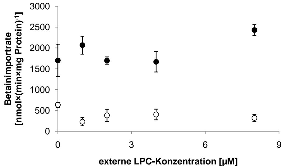
Abbildung 3.11: Einfluss von LPC auf die BetP-Transportaktivität in POPG-reichen Proteoliposomen. Lipidzusammensetzung der Vesikeln: 1/3 E. coli -Lipide, 2/3 synthetisches POPG. Externer Puffer: 20 mM NaCl, 25 mM NaPi pH 7,5, 0,1 osmol/kg. Interner Puffer 0,1 M KPi pH 7,5. Die K + -Konzentration im Proteoliposomenlumen wurde durch das Variieren der externen Osmolalität eingestellt und betrug ca. 180 mM (○) oder ca. 480 mM (●). Dargestellt sind die Mittelwerte von jeweils fünf Messungen mit Standardabweichungen.
