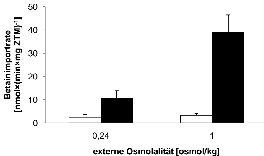
Abbildung 3.1: BetP-Transportaktivität in \text{K}^+ -verarmten C. glutamicum DHPF (pBetP)-Zellen in Abhängigkeit der externen Osmolalität und \text{K}^+ -Supplementation. Die Zellen wurden vor der Betainzugabe 10 min bei 30 °C ohne \text{KCl} (□) oder mit 2,5 mM \text{KCl} (■) inkubiert. Externer Puffer: 0,1 M \text{NaCl} , 25 mM \text{NaPi} pH 8, 0,24 osmol/kg. Die Osmolalität des externen Puffers wurde mit Sorbit eingestellt. Die Transportmessung wurde durch die Zugabe von 0,25 mM radioaktiv markiertem Betain gestartet und 90 s lang verfolgt. Dargestellt sind die Mittelwerte von jeweils drei Messungen mit Standardabweichungen.
