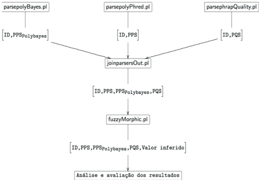
Fig. 2. Síntese da estrutura funcional do modelo de mineração de dados (etapas C, D e E).
