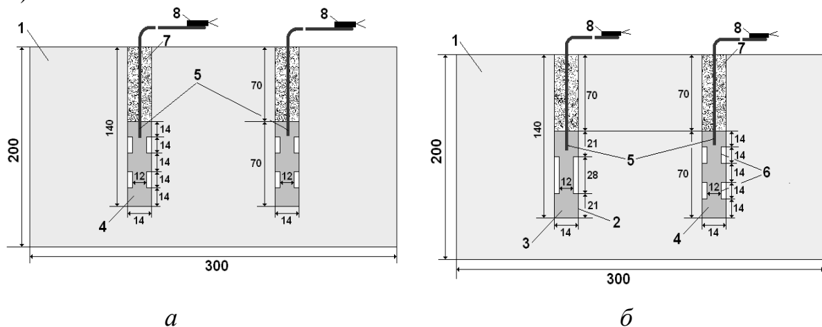
Рис. 2. Схема формирования зарядов ВВ в песчано-цементных моделях в форме параллелепипедов: 1 – песчано-цементная модель; 2 – зарядная полость; 3 – заряд ВВ переменного сечения с одним заужением; 4 – заряд ВВ переменного сечения с двумя заужениями; 5 – детонирующий шнур; 6 – заужения в цилиндрических зарядах; 7 – забойка; 8 – электродетонатор
