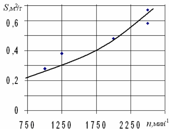
Рис. 1. Залежність удельної поверхності продуктів струйного измельчення шлака від частоти обертання ротора класификатора, шлак вихідний, крупність 3-0 мм
