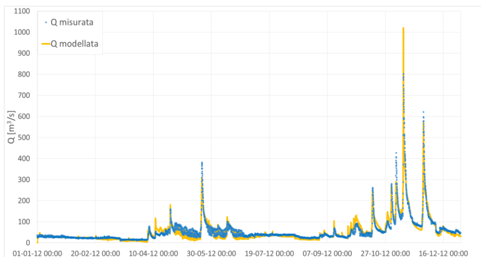
Figura 2. Confronto tra i risultati del modello idrologico e i dati misurati a Bassano del Grappa per l'anno 2012.
