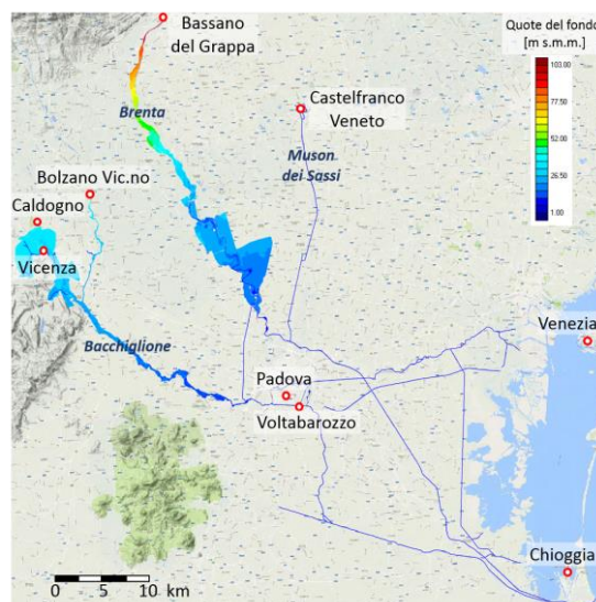
Figura 1. Dominio di calcolo del modello idrodinamico. I colori indicano le quote del fondo.
