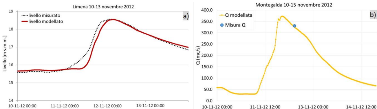
Figura 3. Confronto tra a) livello misurati e modellati dal modello idrodinamico a Limena e b) tra la portata misurata e modellata dal modello idrodinamico a Montegalda, durante l’evento di piena del 12 novembre 2012.
