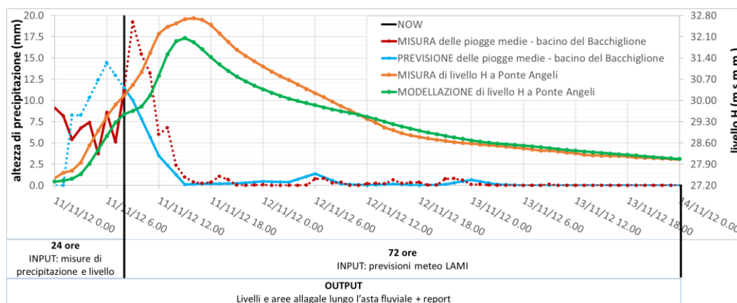
Figura 4. Esempio di prestazione della catena modellistica applicata in corso d'evento.
