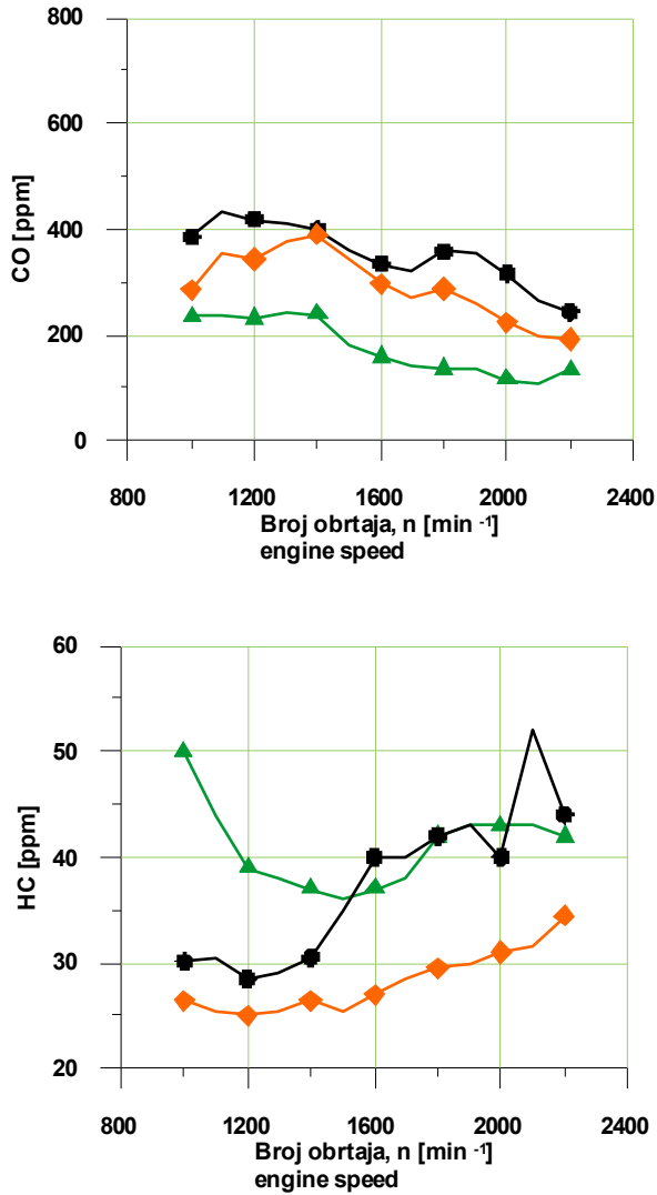
Slika 6b: Emisija najizraženijih štetnih komponenti (CO, HC) u ispušnim plinovima motora SUI za slučaj korištenja fosilnog i biodizela, te mješavine B50 pri kutu ubrizgavanja goriva od 21^\circ KV prije GMT
