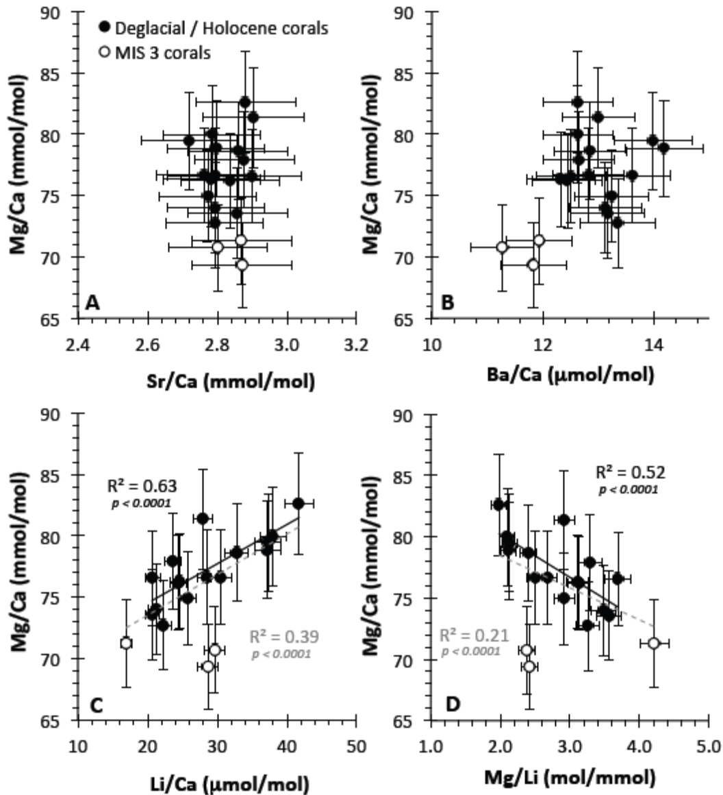
Figure 10. Gutjahr et al. Chemical Geology
