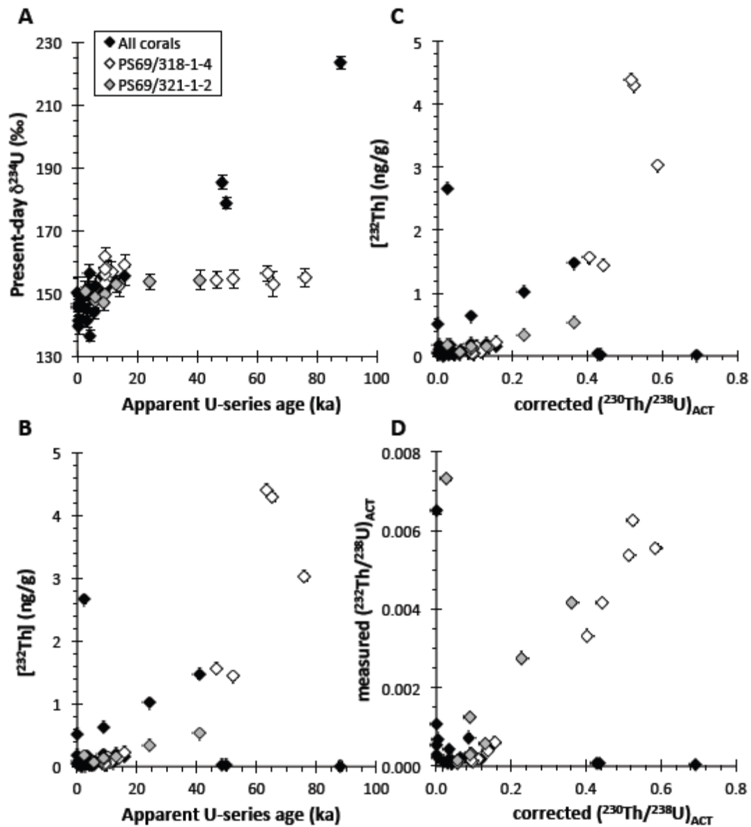
Figure 7. Gutjahr et al. Chemical Geology
