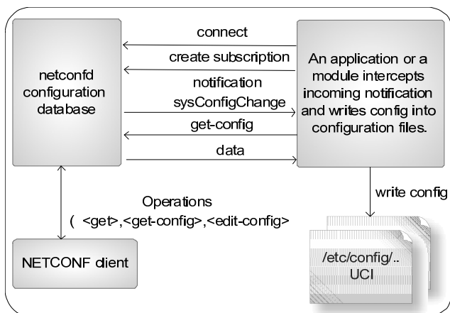
Fig. 3. NETCONF usage
