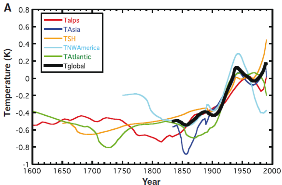
Abbildung 1. Temperatur Rekonstruktion für verschiedene Regionen. Die schwarze Kurve zeigt einen geschätzten globalen Mittelwert. SH=Südliche Hemisphäre (Oerlemans, 2005, Science 308).
