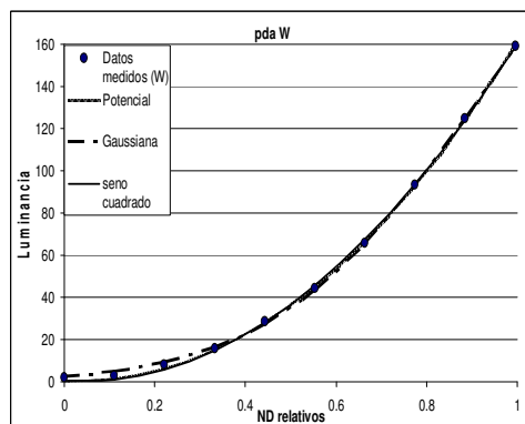
Figura 1: Gráfica con el ajuste potencial y con otras dos curvas de mejor ajuste para la Pda
