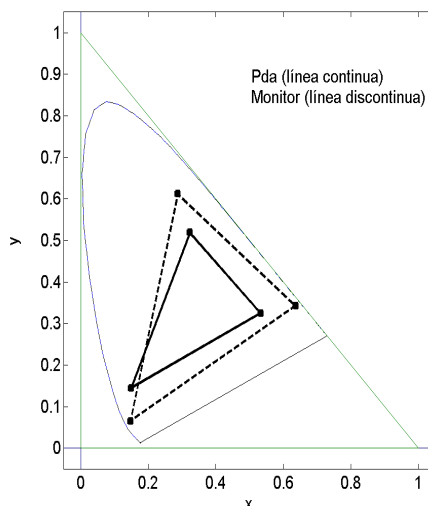
Figura 2: Triángulo de primarios para la pda y el monitor LG en el espacio CIExy
