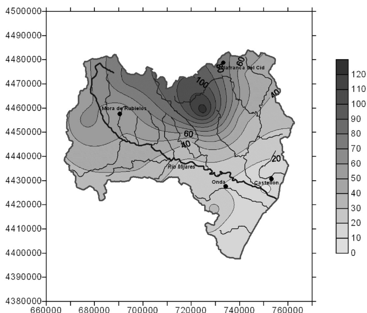
FIGURA 13. Escorrentía global (mm) del Sistema Hidrográfico del río Mijares-La Plana bajo un escenario climático configurado por un aumento térmico de +1°C y una reducción de las precipitaciones del 5 %.
