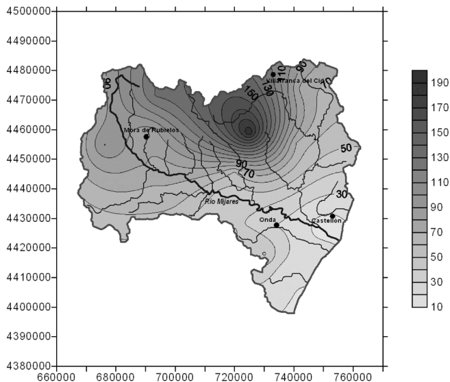
FIGURA 12. Escorrenías medias anuales sobre el Sistema Hidrográfico del río Mijares-La Plana (1950-2000). El valor medio anual es de 76 mm.
