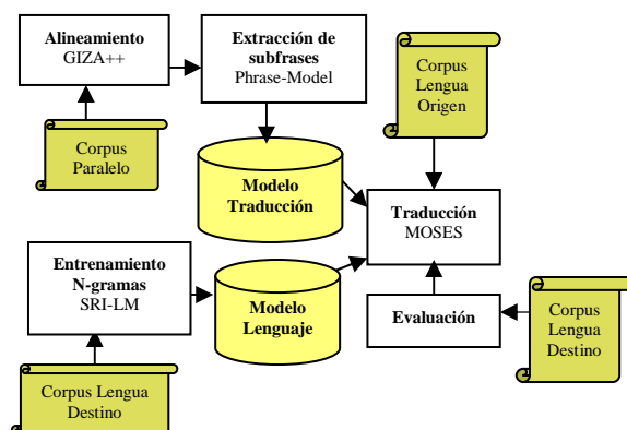
Figura 2: Arquitectura completa del sistema de traducción basado en subfrases
