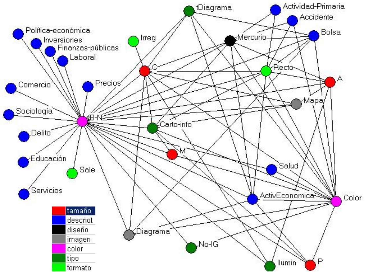
Ilustr. 10: Mapa de asociación de variables (grado 10)
