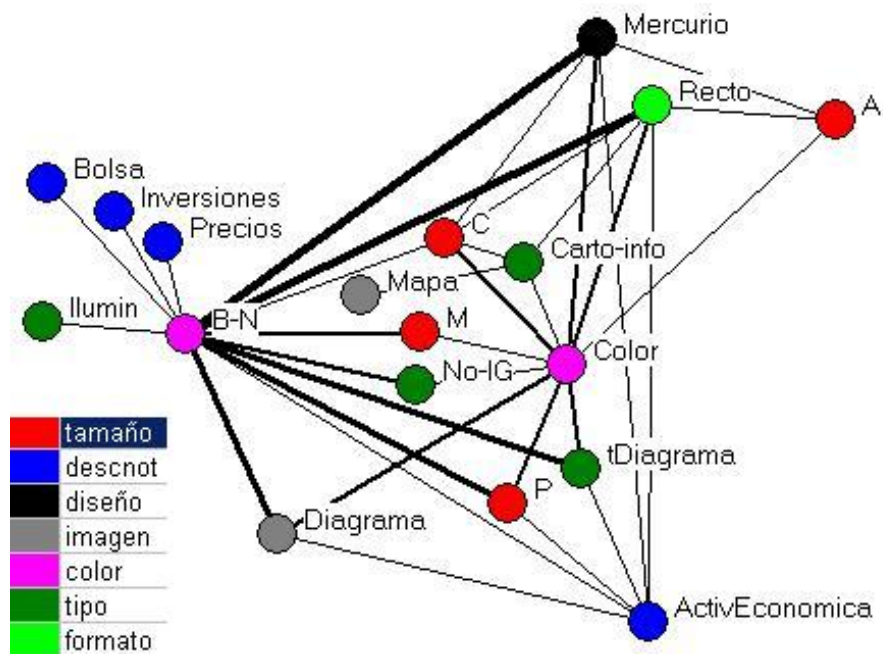
Ilustr. 9: Mapa de asociación de variables (grado 20)
