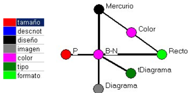
Ilustr. 11: Mapa de asociación de variables (grado 80)
