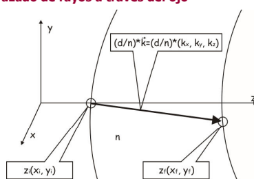
Figura 2. Esquema de obtención del camino óptico entre superficies
