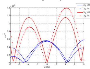
Figura 6. Componentes absolutas astigmáticas x/y y comáticas x/y de la potencia refractiva para el ojo modelado con un cristalino inclinado un ángulo 0^\circ y 3^\circ .
