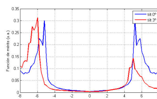
Figura 5. Función de mérito en eje x para el ojo modelado con un cristalino inclinado un ángulo 0^\circ y 3^\circ .
