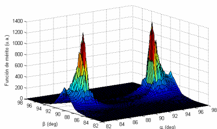
Figura 3. Valores de la función de mérito para ángulos de incidencia vertical y horizontal en el rango [-8^\circ, 8^\circ] .
