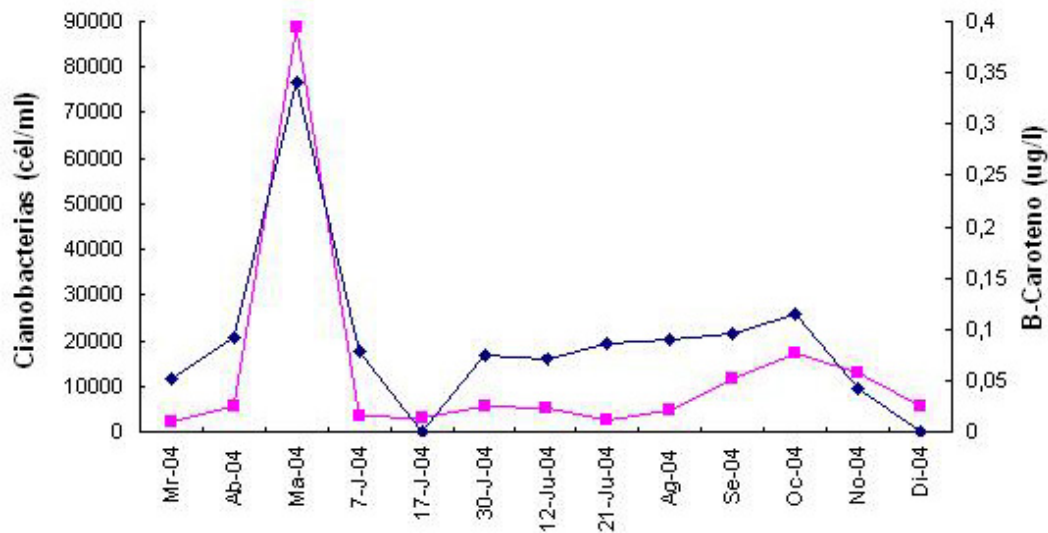
Figura 4. Perfiles zeaxantina-cianobacterias y \beta -caroteno-cianobacterias correspondientes al pantano Choça Queimada, profundidad superficie. En abcisas se recogen las fechas de muestreos.
