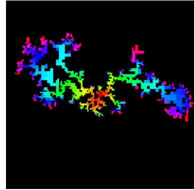
DLA
