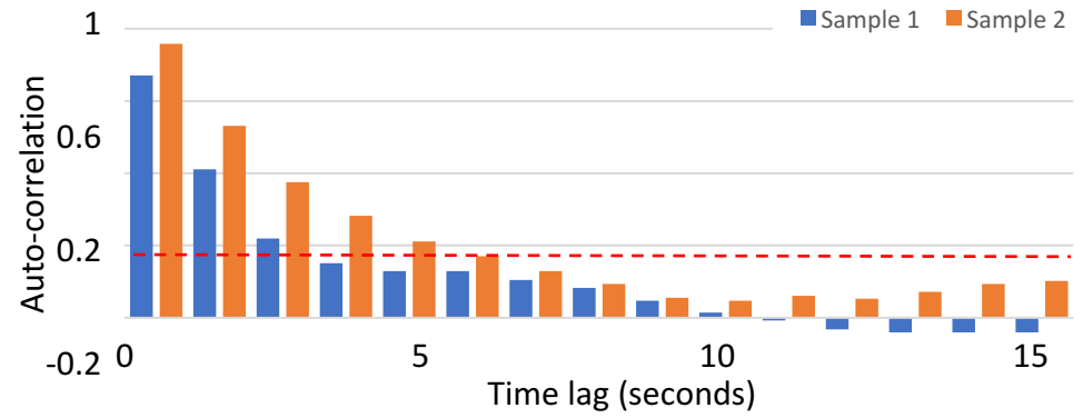
c) ACF
