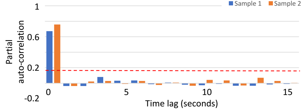
d) PACF
