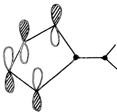
HOMO
