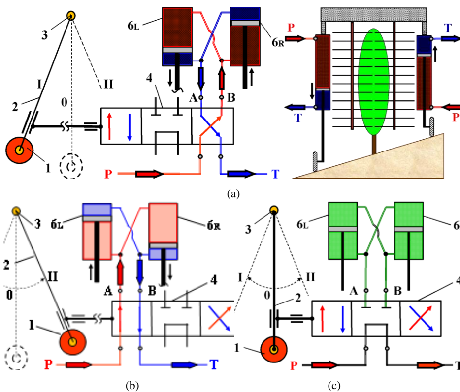
Slika 1. Sistem nivelacije: (a) podizanje desnog i spužtanje levog točka pri radu na nagibu (b) obrnut proces poravnavanja i (c) neutralno stanje na vodoravnom terenu, [21].
