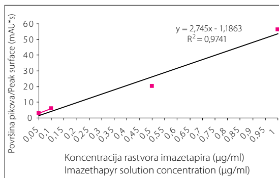
Slika 2. Linearnost detektora
