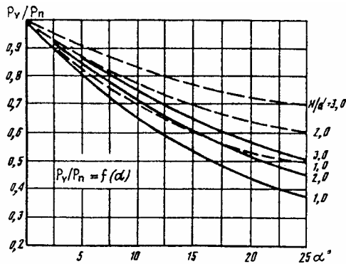
Sl. 5. Uticaj nagiba i odnosa H/d na veličinu srednjeg koeficijenta relativne neravnomernosti za stalne uglove mlaznice i to:
