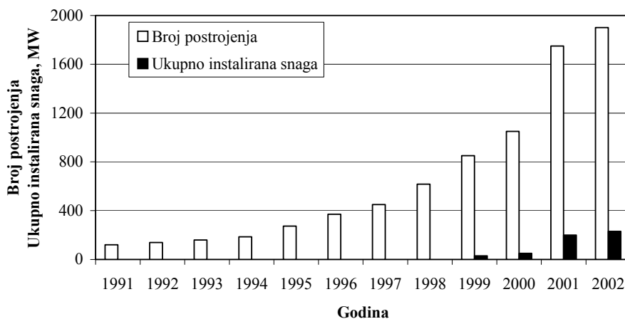
Slika 1 Promena broja postrojenja i ukupne instalisane snage na biogas u poljoprivredi Nemačke
