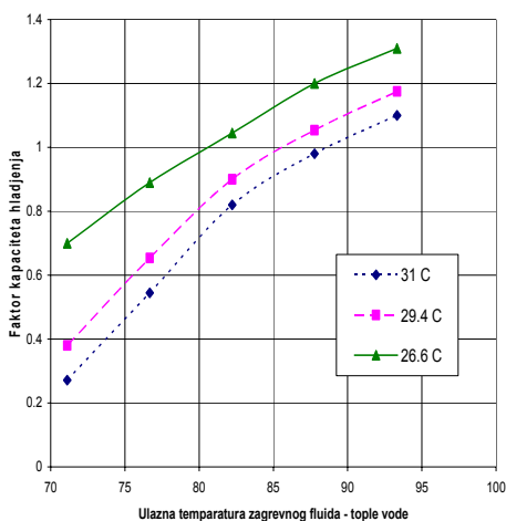
Slika 1. Zavisnost promene kapaciteta hlađenja od ulazne temperature zagrevnog fluida
