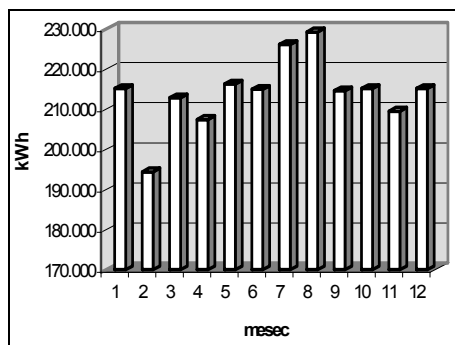
Slika 7. Potrebna energija gasa za kogeneraciju
