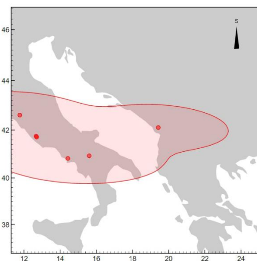
Slika 33 Prostiranje Avellino tefre s mjestima pronalaska. Preuzeto iz RESET baze podataka.
