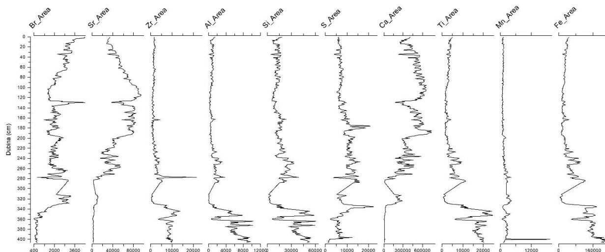
Slika 17 Varijacija odabranih elemenata duž jezgre M2 dobivenih \mu -XRF analizom. Koncentracije su izražene kao cps (counts per second) na X osi.
