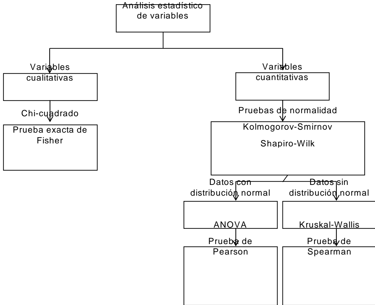
Figura 3. Algoritmo del análisis estadístico de variables
