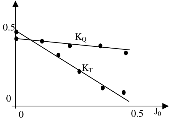
Fig. 6. Propeller parameters
