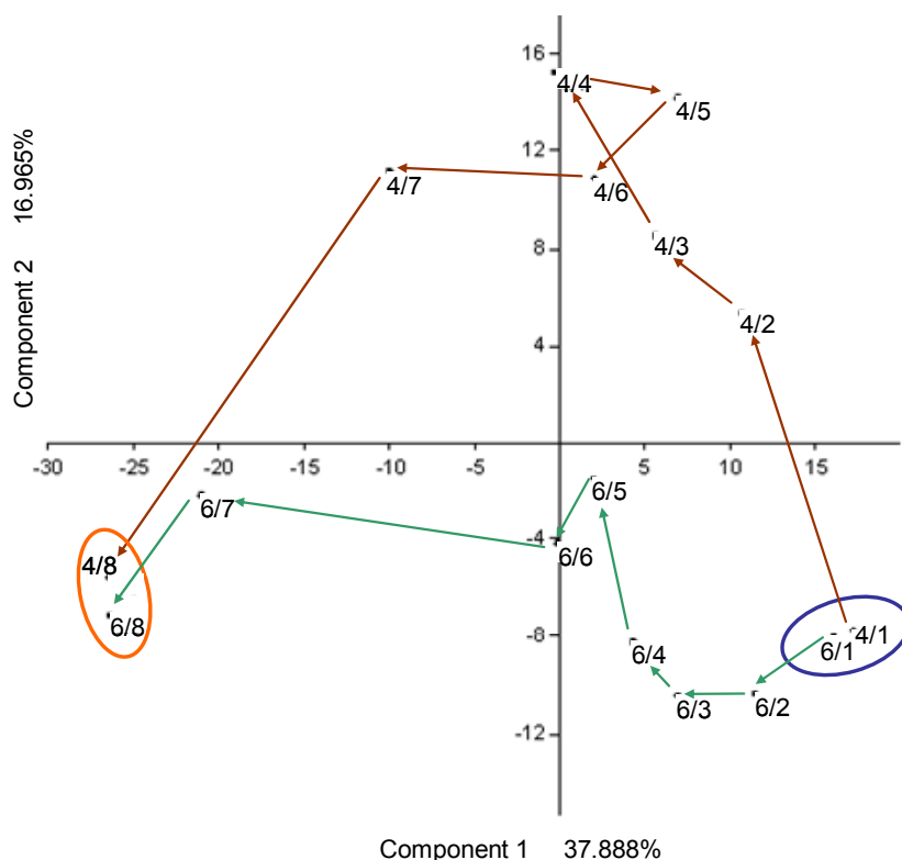
4. ábra. A három markertípus (TR-F, foszfolipid-zsír-sav és respiratórikus kinon) alapján végzett főkomponens-analízis konszenzus-eredménye a felfűtéses kísérletben. A kék kör a mezofil kiindulási állapotot, a piros a kísérlet végi termofil állapotot jelöli. A barna nyilak a 4-es reaktor (hirtelen felfűtés), a zöldek a 6-os reaktor (fokozatos felfűtés) közösségének szukcessziós útját követik.
