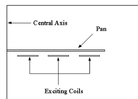
Рис. 9. Ескіз двовимірної розрахункової моделі системи «індуктор – посуд» [14]
