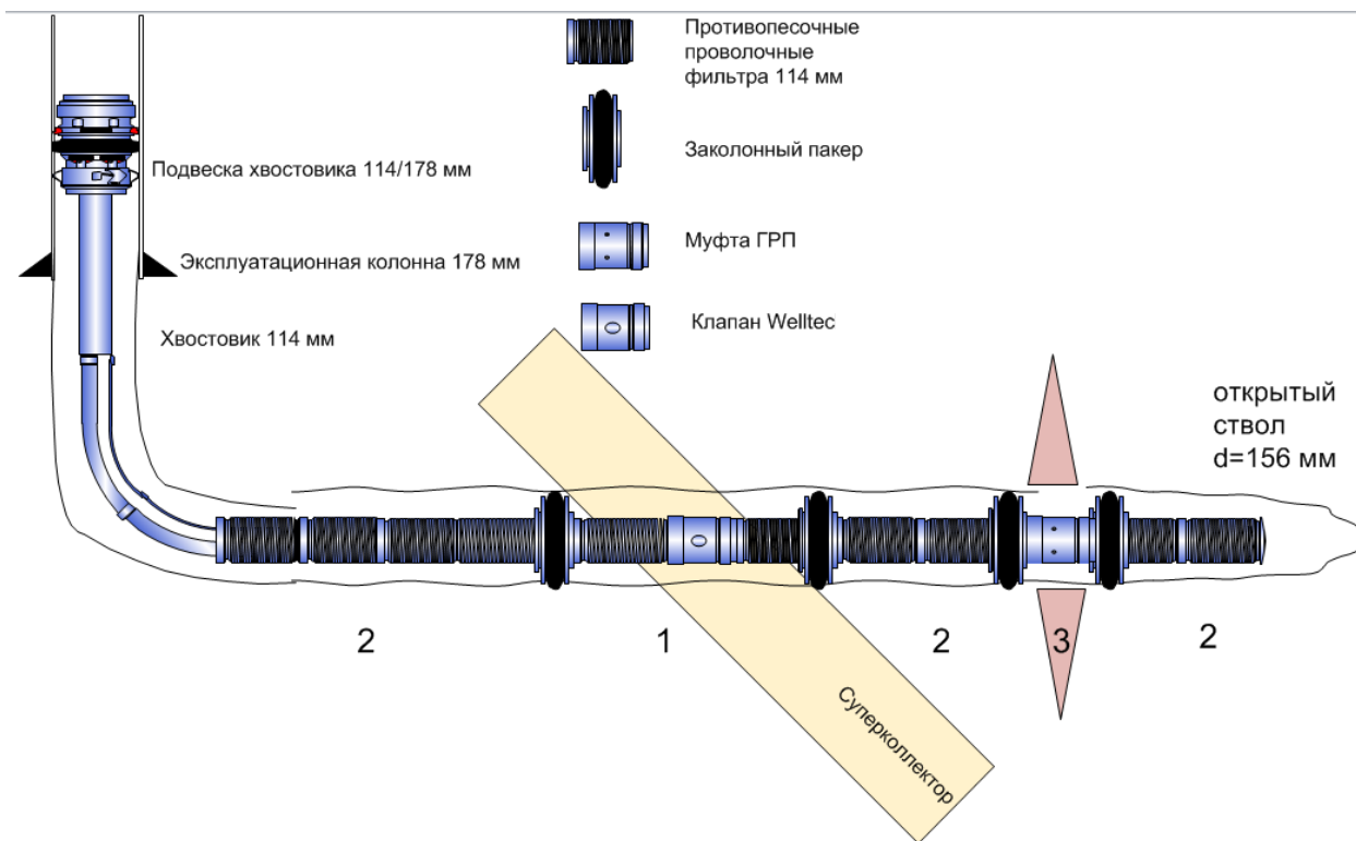
Рисунок 3 – Комбинированное заканчивание [10]
