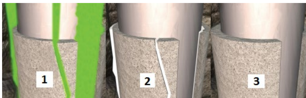
Рисунок 10 – Восстановление целостности цементного кольца потоком углеводорода
